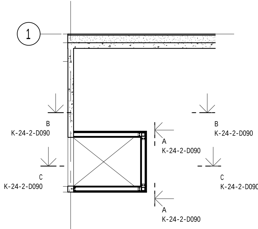
PLAN STÅLSEKTIONER HISS 1 : 50
