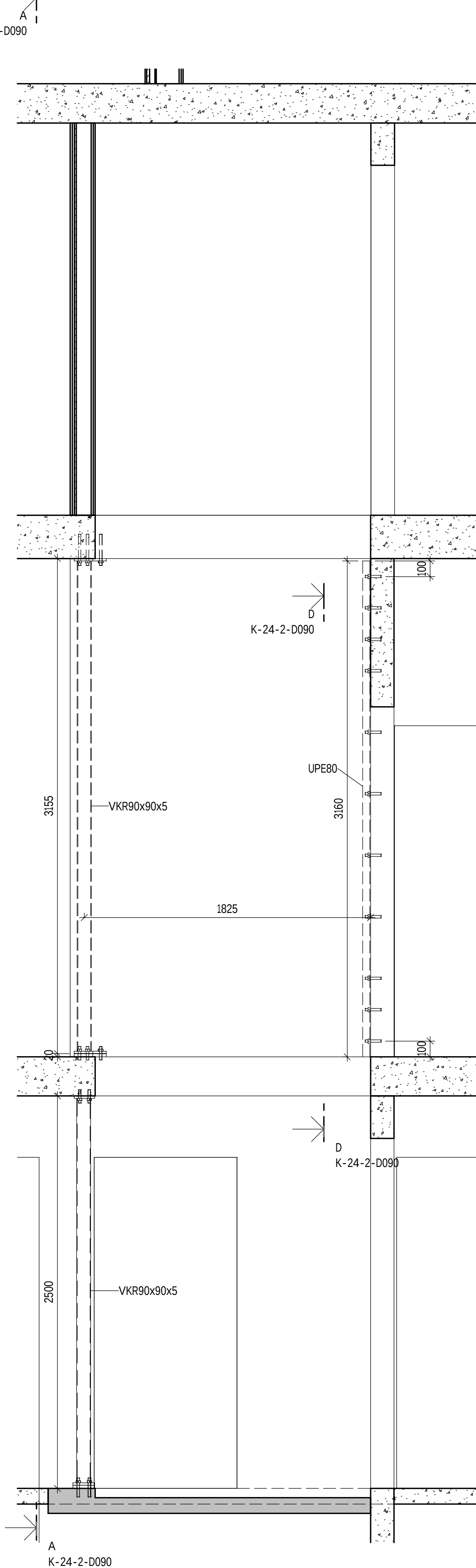
C-C 1 : 20
