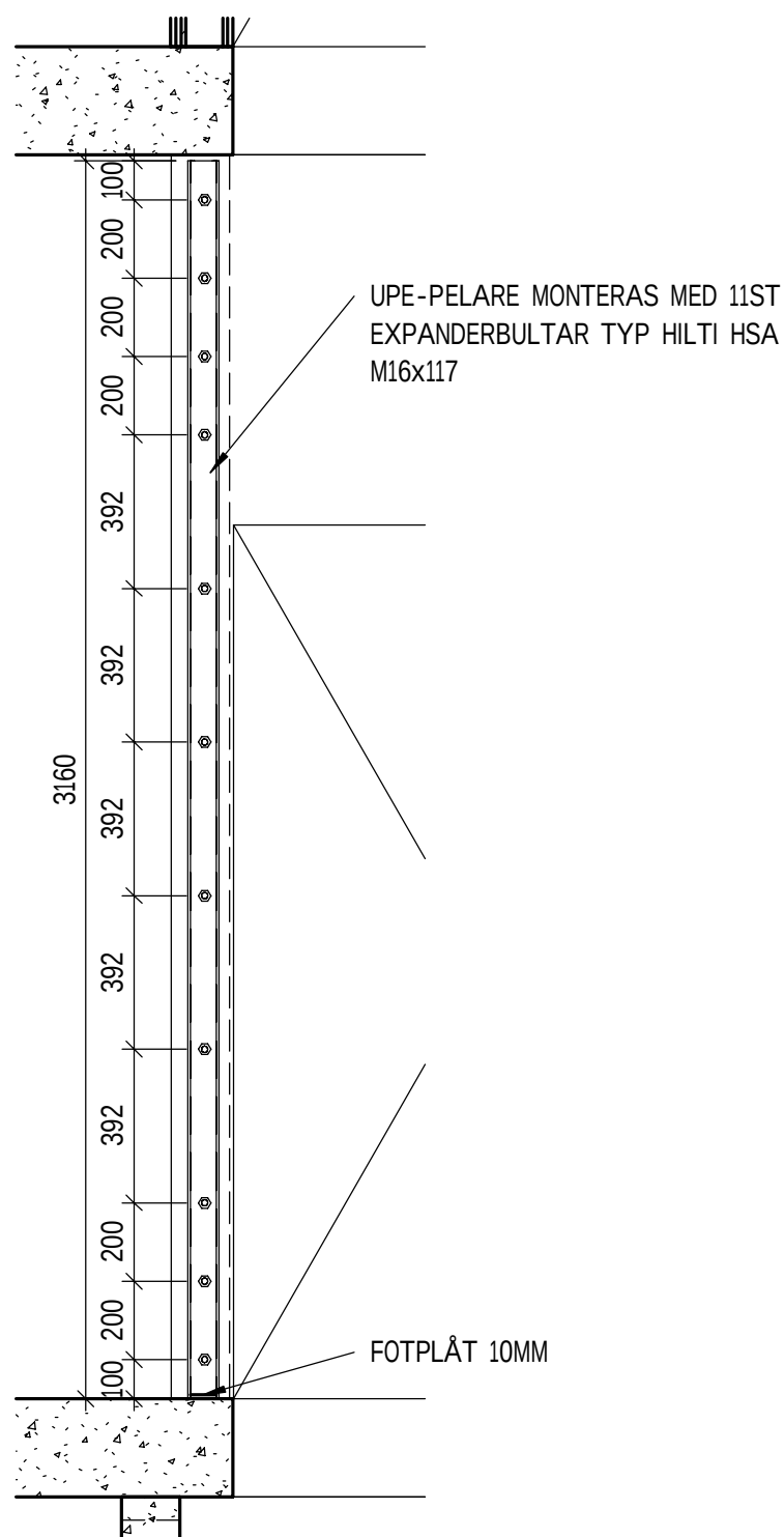
D-D 1 : 20
